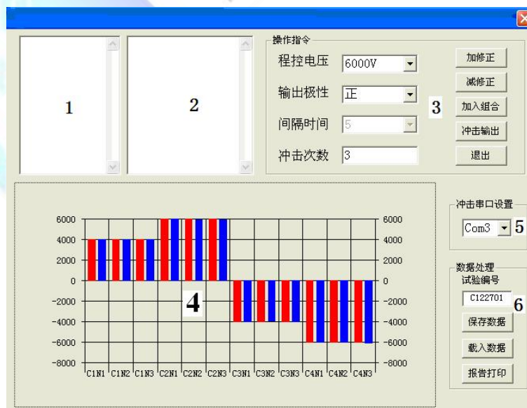
图 4 计算机控制基础版图示
