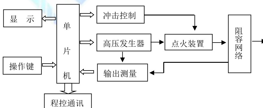
图 1 原理框图
