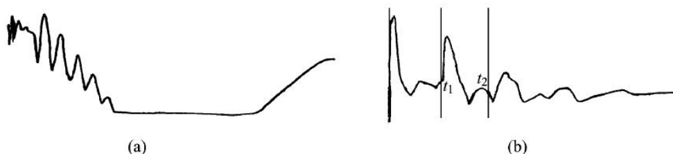
(a) CVF 法实测波形；(b) CVF 法电缆另一端实测波形
