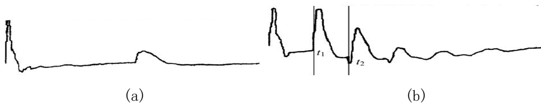
(a) 冲击电压为 25kV 实测波形；(b) 冲击电压为 25kV 压缩波形
