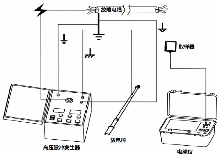
一 体 式（高压脉冲发生器+电缆仪）
