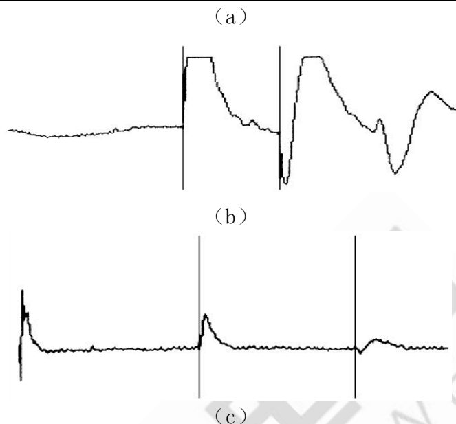
(a) 25kV 实测波形；(b) 25kV 扩展波形；(c) 25kV 另一端实测波形
