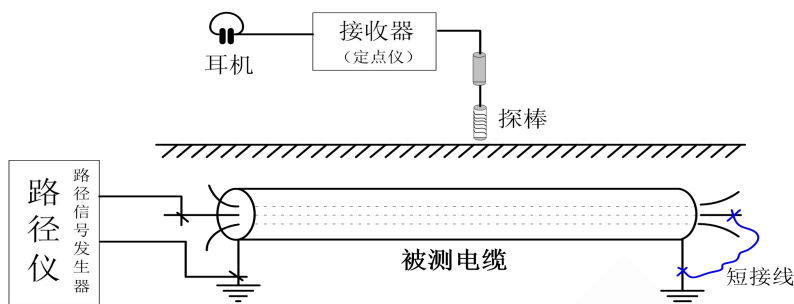
超长电缆或断线电缆路径探测接线示意图
