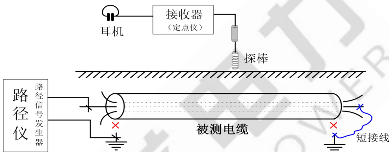
特殊路径探测接线示意图
