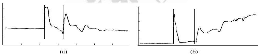
(a) 电流法实测波形；(b) 电压法实测波形
