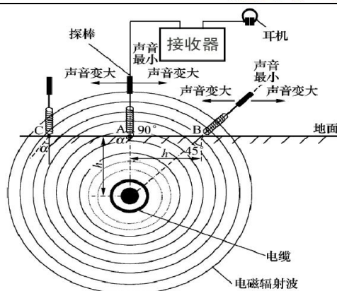
探棒放置示意图
