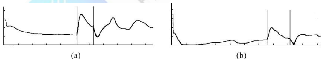
图 7 福州自来水公司电力电缆实测波形
