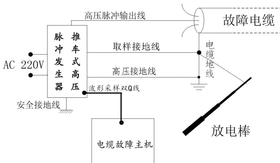
一 体 式（推车式高压脉冲发生器+电缆仪）
