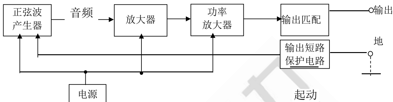
路径仪工作原理框图
