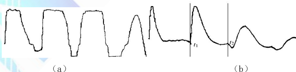
(a) 冲击电压为 20kV 实测波形；(b) 减小输入幅度后的波形
