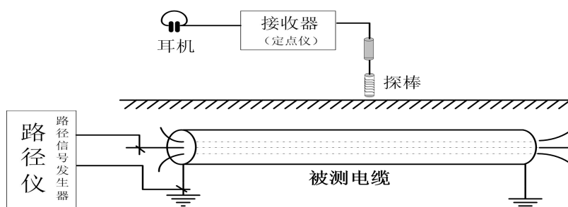
一般路径探测连线示意图
